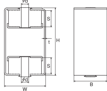
吊防振ゴムセット ダブル(W5/8・3/4)
