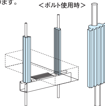
〈ボルト使用時〉
