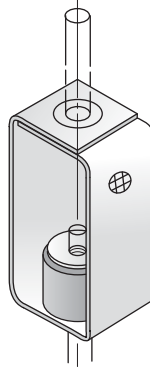
シングル仕様(S) 施工状態
