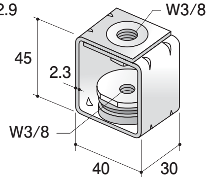
吊防振ゴムセット ミニ ナット付
