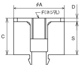
吊防振ゴム(W3/8・1/2)
