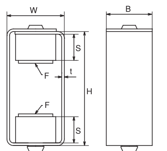
吊防振ゴムセット ステンレス ダブル (W3/8・1/2)
